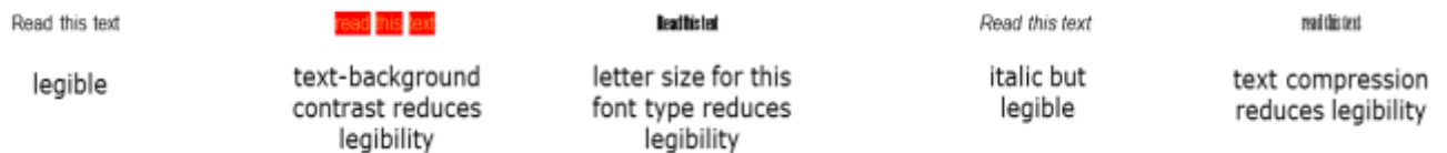
Figuur 4: Leesbaarheid
